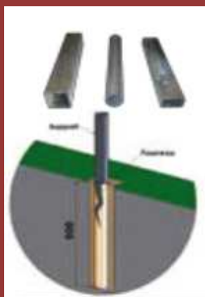
Fourreau en acier galvanisé L. 500 mm Pour tube 80 x 80 Pour tube 80 x 40 Pour tube diam.60
